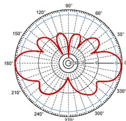
H-Plane Pattern
